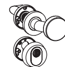
Schutz-Rosetten-Garnitur R1/ZA Außen Knopf R1 und Schutzrosette + Kernziehschutz. Innen Drückerrosette + PZ Rosette
