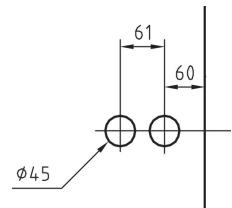
Bohrungen Schlosskasten Bores glass-door lock
