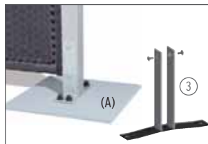
Standträger für Hohlpfosten (3) zum Aufschrauben oder einen Standard-Anker für 7 x 7er Pfosten (Erdverbau).
